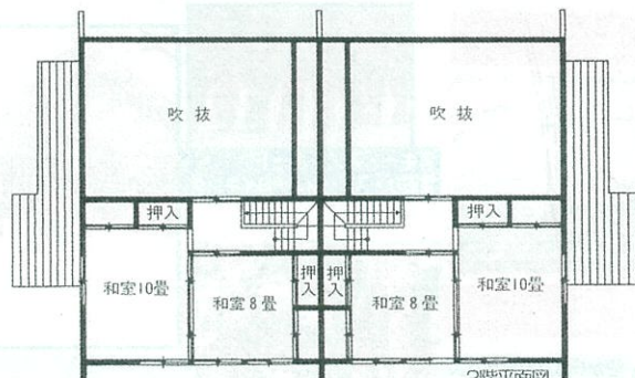
2階平面図
